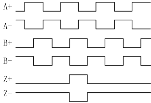
图 4 ABZ 信号
