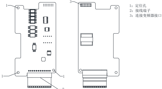
图1 PG11S 外观（3.7kW 及以下机型适配）
