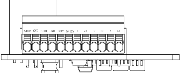
图3 端子丝印示意图
