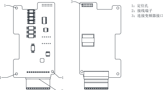
图2 PG21S 外观（5.5kW 及以上机型适配）
